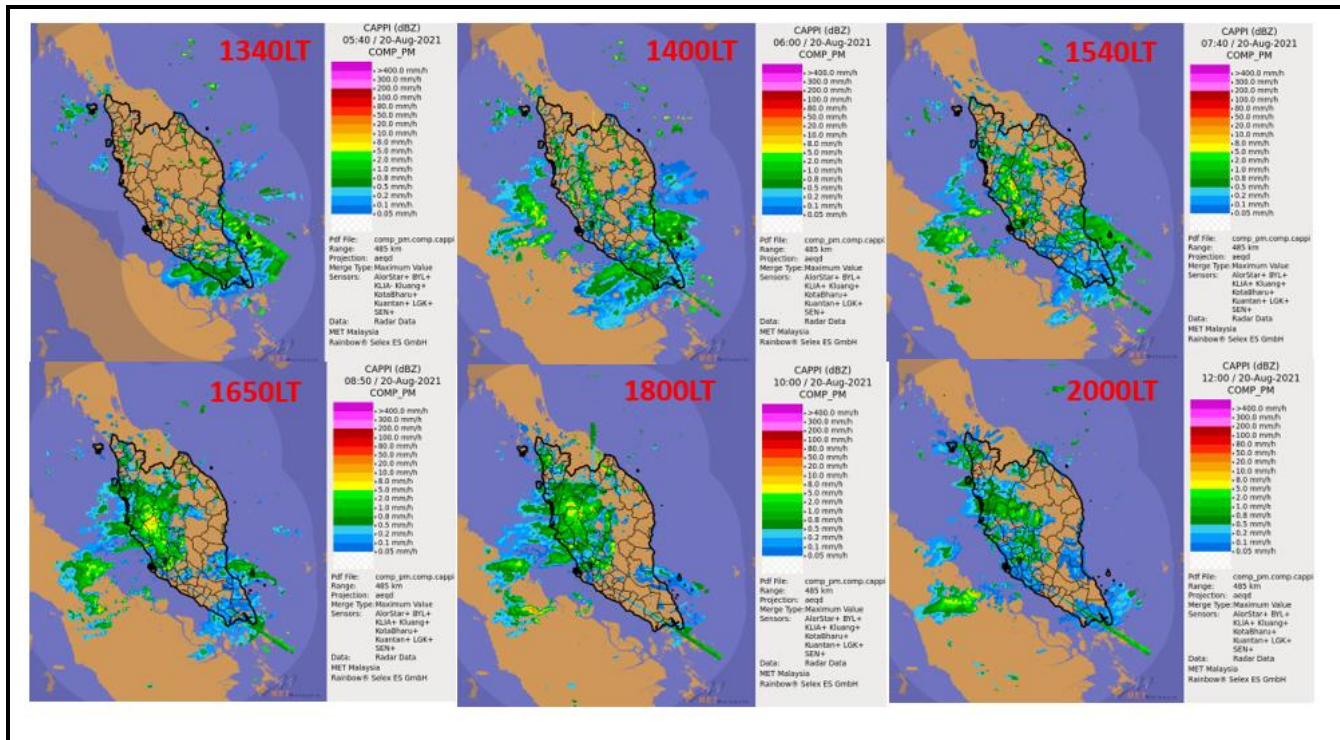
Rajah 2: Pencerapan imej radar pada 1:40 tengah hari hingga 8:00 malam pada 20 Ogos 2021
