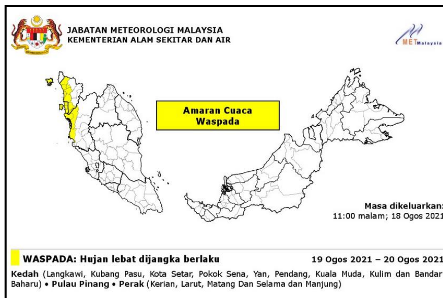
Rajah 3: Amaran Cuaca Waspada yang dikeluarkan pada 18 Ogos 2021 untuk tempoh berkuat kuasa pada 19 hingga 20 Ogos 2021
