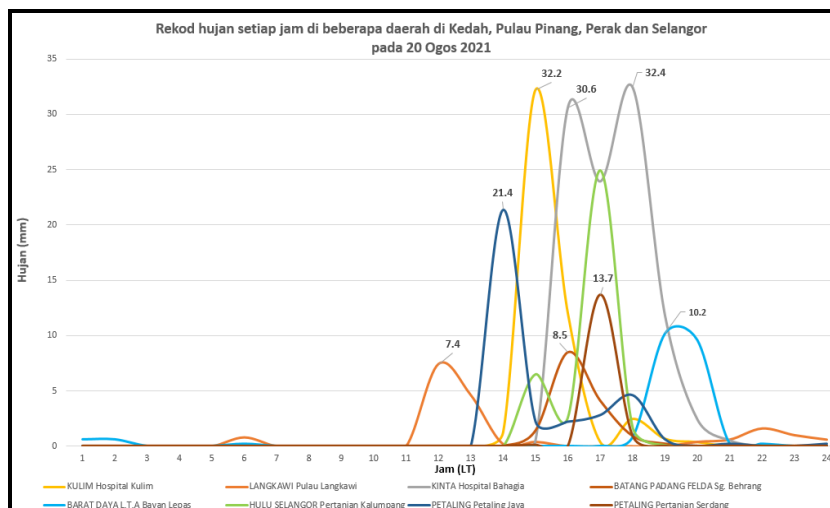
Rajah 1: Data Hujan Setiap Jam di Stesen Meteorologi di Kedah, Pulau Pinang, Perak dan Selangor pada 20 Ogos 2021
