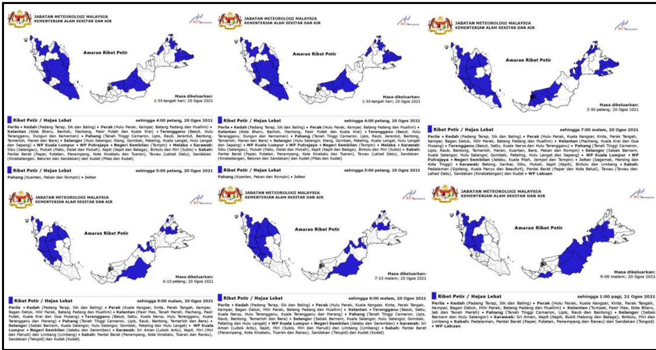
Rajah 4: Siri Amaran Ribut Petir yang dikeluarkan untuk negeri Kedah, Perak dan Selangor pada 20 Ogos 2021
